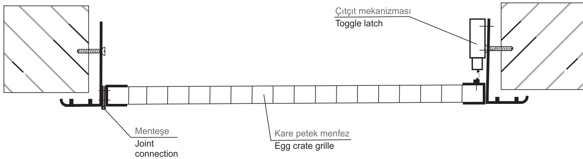
Çıtçıtlı çerçeve montaj şekli Assembly details of frame with toggle latch
