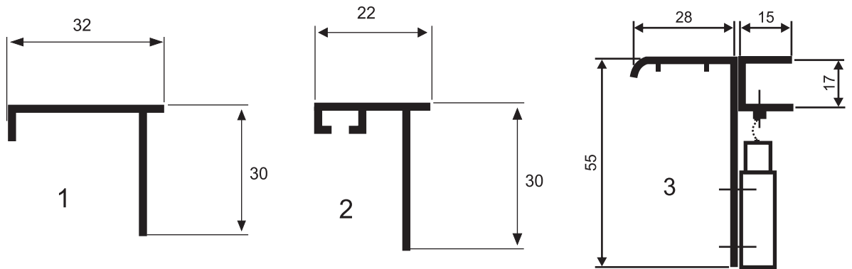
Standart çerçeve / Standart frames
